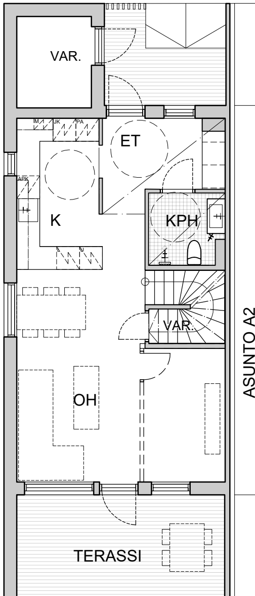
POHJAPIIRROS 1 KRS.
