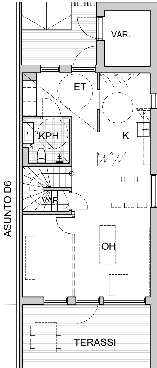
POHJAPIIRROS 1 KRS.
