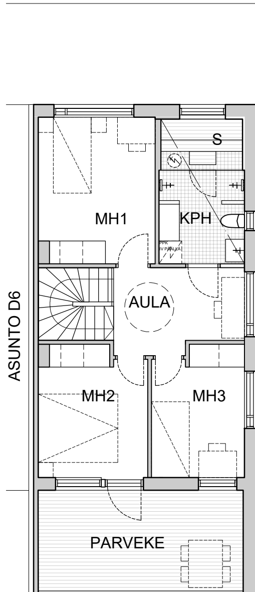
POHJAPIIRROS 2 KRS.
