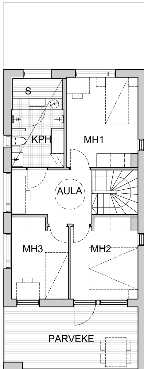
POHJAPIIRROS 2 KRS.
