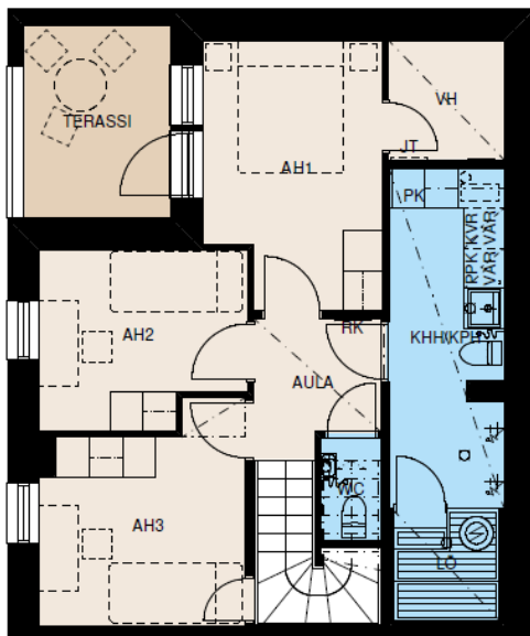
1. KERROS
