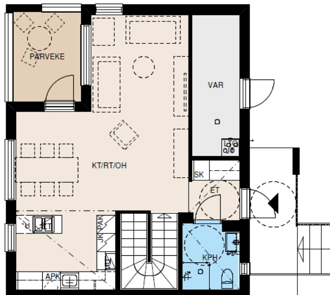
2. KERROS
