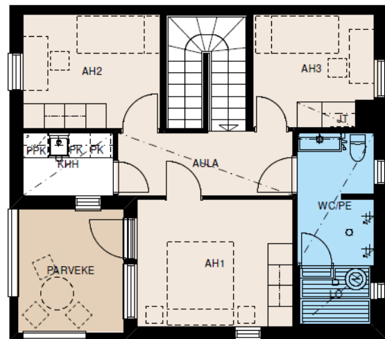
2. KERROS
