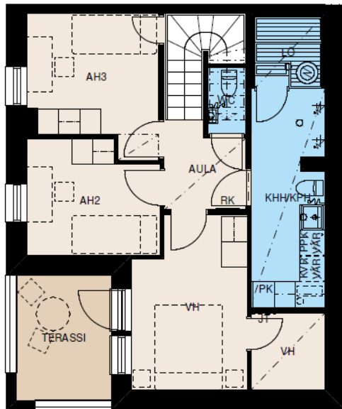
1. KERROS
