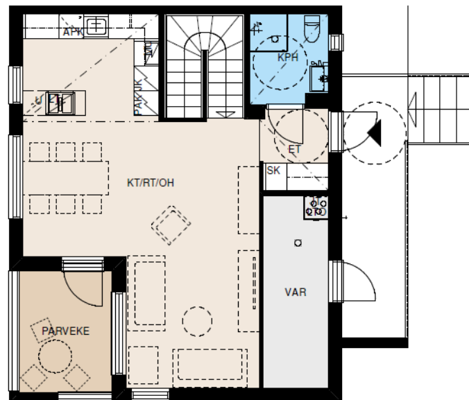
2. KERROS
