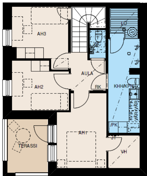
1. KERROS
